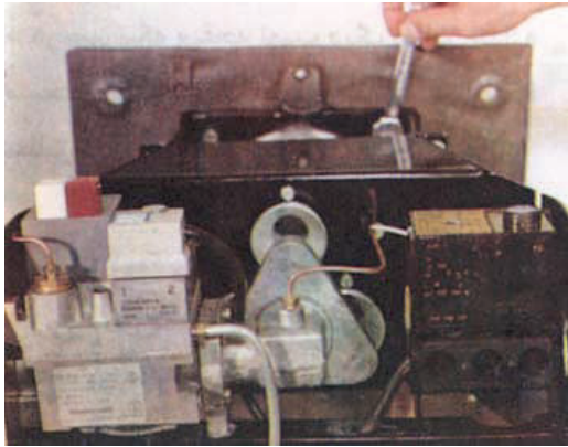
شکل ۳۰-۲- نصب مشعل روی دیگ
