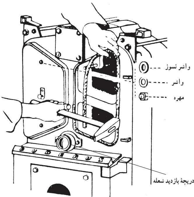
شکل ۱۴-۲- بستن دریچه بازدید شعله
