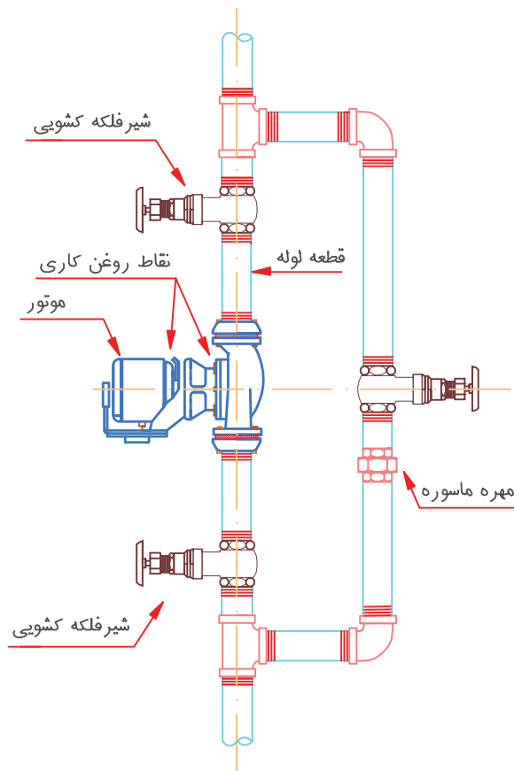
شکل ۱۹-۲- پمپ سیرکولاتور با مدار بای پاس
